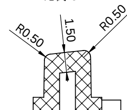
剖面 A-A 比例 5:1
