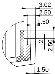
局部视图 C 比例 2.4 : 1
