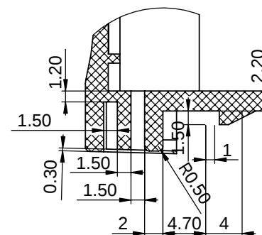
局部视图 D 比例 2.4 : 1
