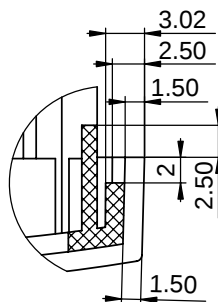
局部视图 C 比例 2.4 : 1
