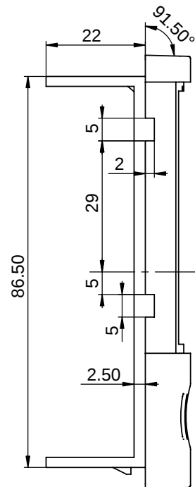
局部视图 C 比例 2.4 : 1
