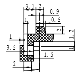
细节 B 比例 5:2
