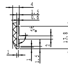
细节 C 比例 6:5
