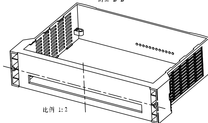
剖面 B-B
