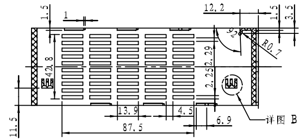
剖面 A-A
