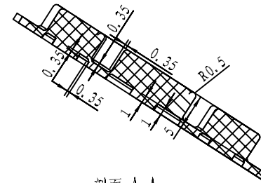
剖面 A-A
