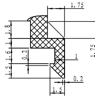
细节 A 比例 6:1
