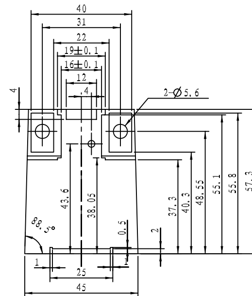
A向视图
