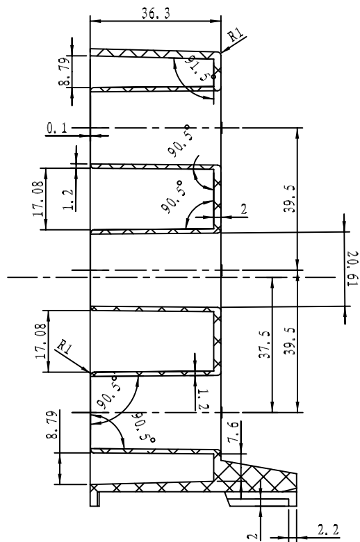
剖面 A-A
