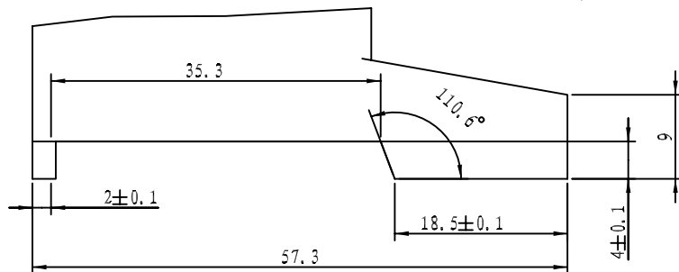
剖面 B-B
