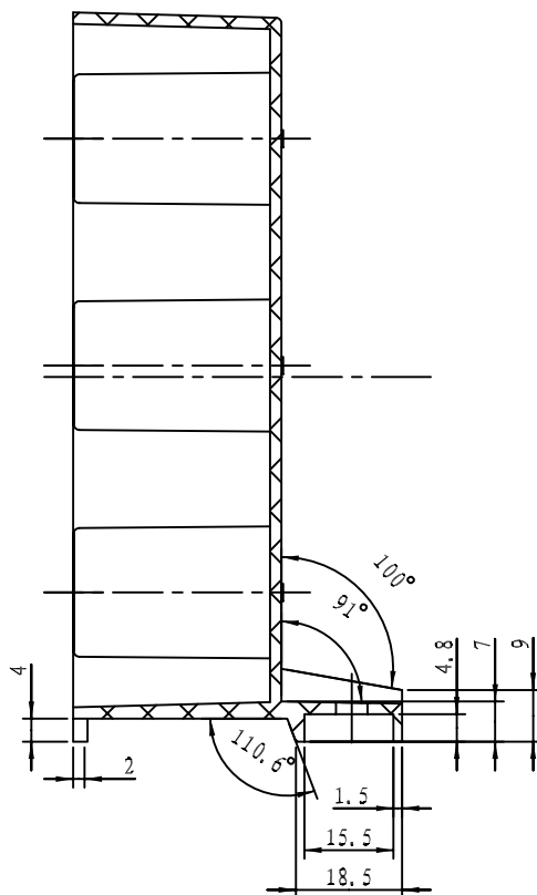
剖面 B-B
