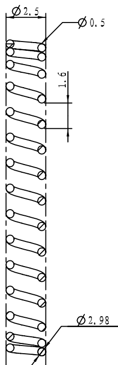
剖面 A-A
