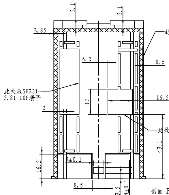
剖面 B-B
