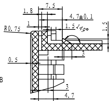
剖面 B-B
