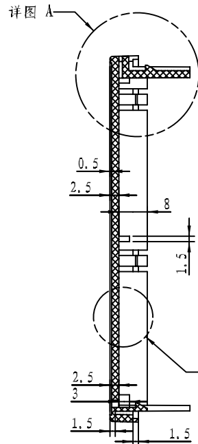
剖面 A-A
