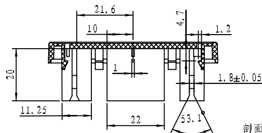
剖面 B-B
