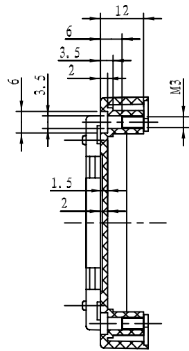
剖面 A-A
