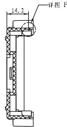
剖面 G-G
