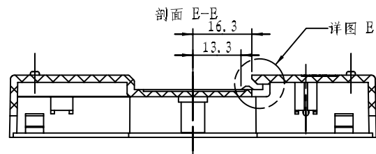
剖面 E-E
