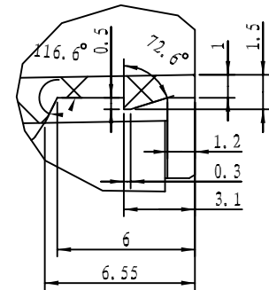
细节 F 比例 5:1
