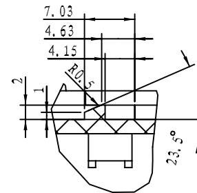
剖面 G-G
