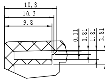
细节 C 比例 3:1
