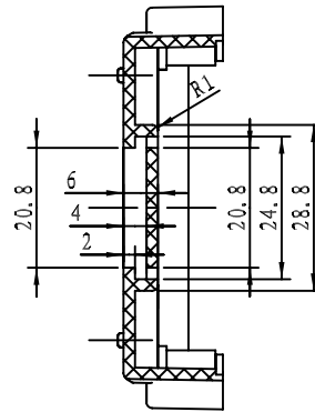
剖面 D-D
