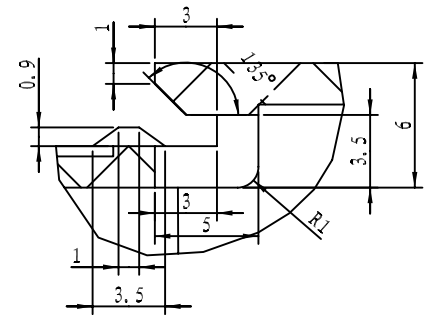
细节 E 比例 4:1
