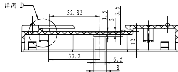
剖面 A-A
