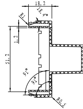
剖面 E-E
