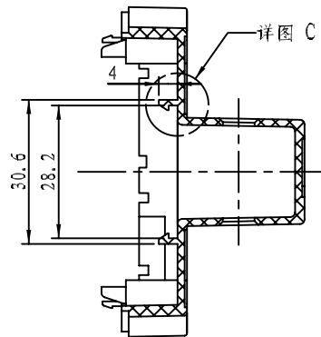
剖面 C-C
