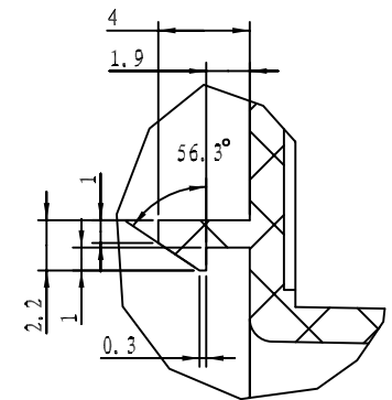
细节 C 比例 4:1
