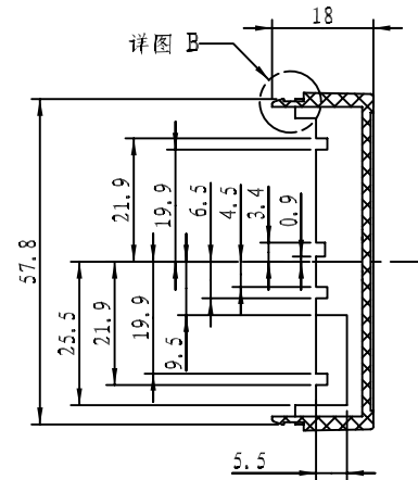
剖面 D-D
