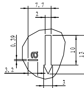
细节 A 比例 2:1
