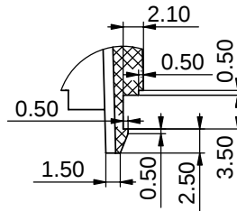
局部视图 C 比例 2:1
