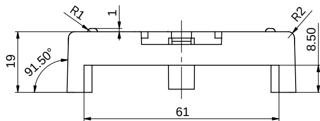
剖面 A-A
