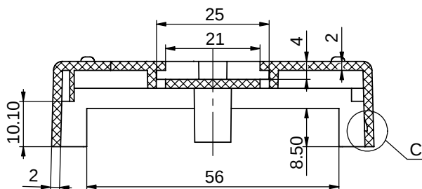
剖面 A-A
