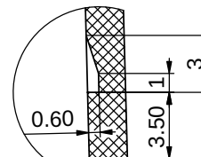
局部视图 C 比例 4:1
