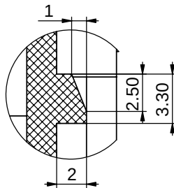
局部视图 E 比例 4:1
