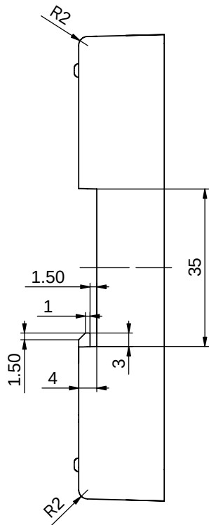
局部视图 E 比例 4:1
