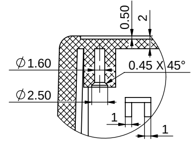
局部视图 E 比例 2.4:1
