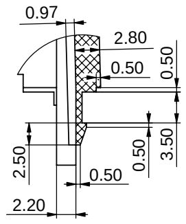
局部视图 D 比例 2.4:1
