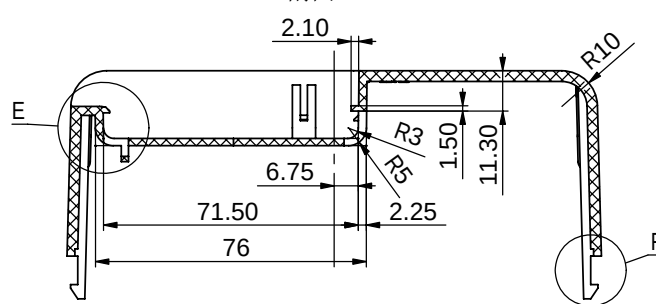
剖面 B-B
