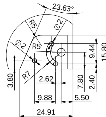
局部视图 D 比例 2:1.5
