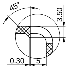
局部视图 G 比例 2:1
