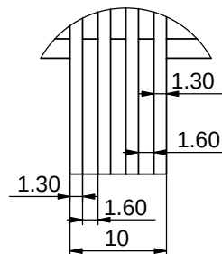
局部视图 I 比例 2:1
