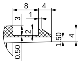
局部视图 H 比例 2:1
