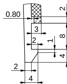
局部视图 F 比例 2:1
