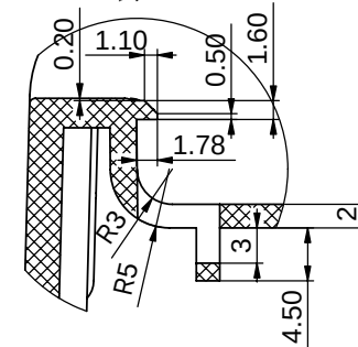
局部视图 E 比例 2:1
