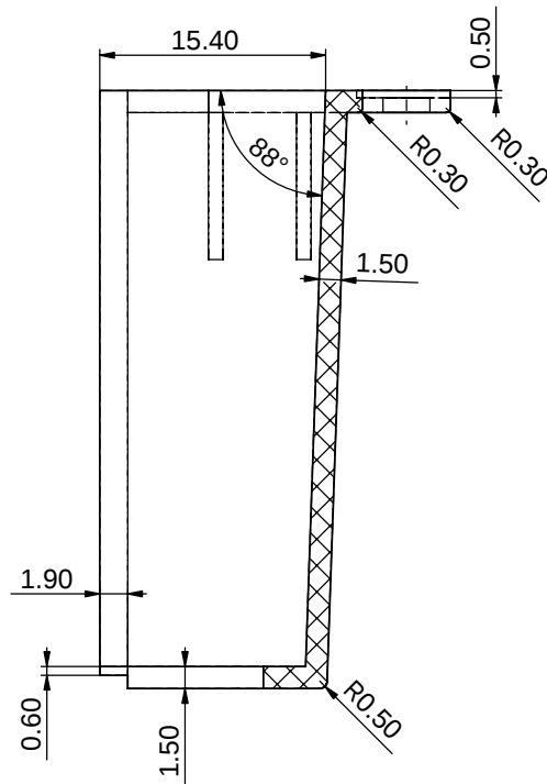
剖面 A-A
