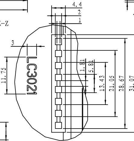
细节 B 比例 2:1
