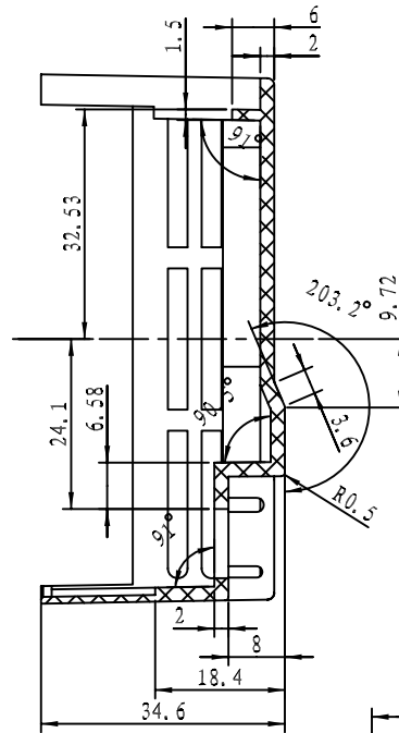
剖面 Z-Z
