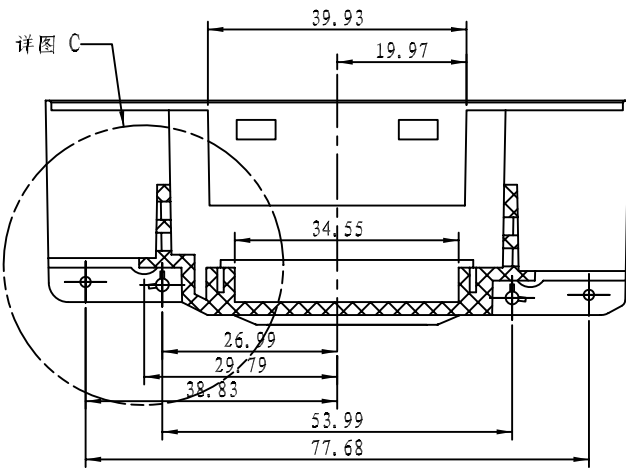
剖面 CY-CY
