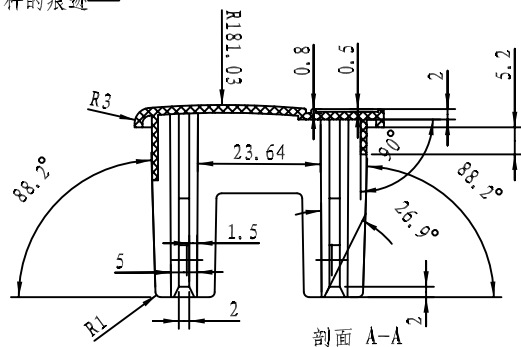
剖面 A-A
