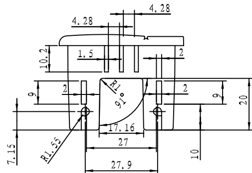
剖面 A-A
