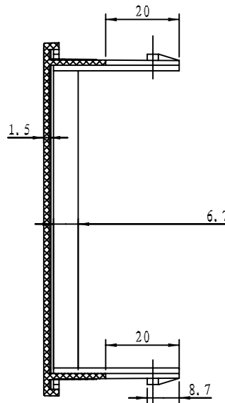
剖面 B-B
