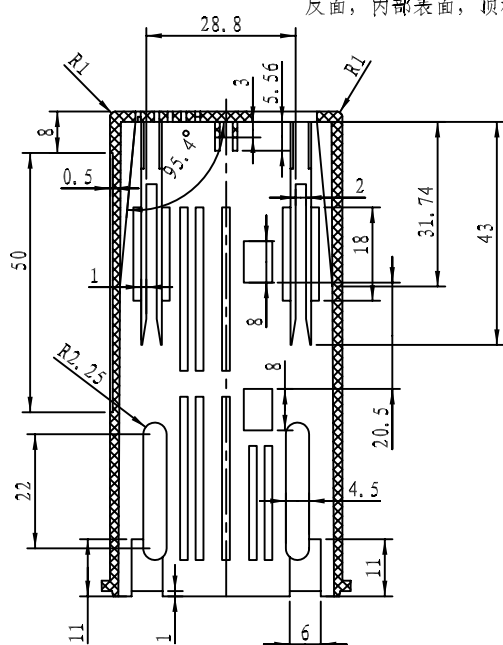
剖面 B-B
