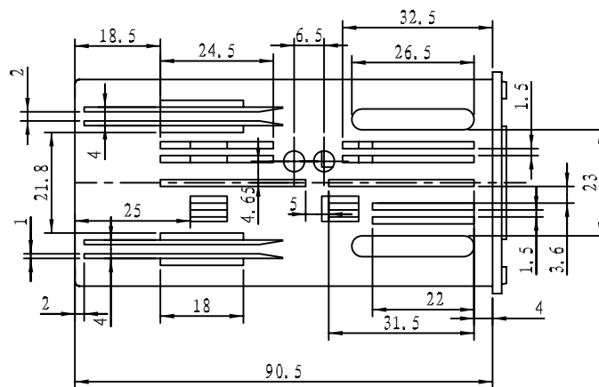
剖面 A-A
