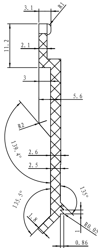
剖面 A-A
