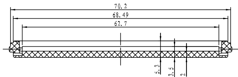
剖面 PZ-PZ
