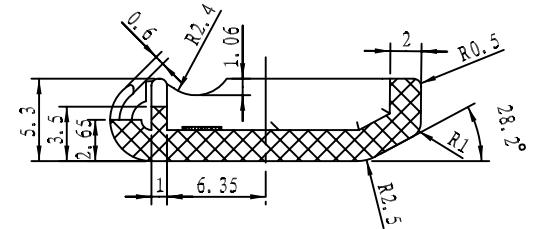
细节 C 刻度 3:1
