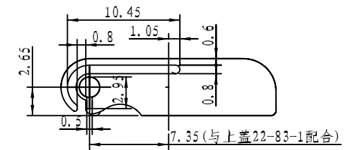
细节 D 刻度 3:1
