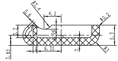
细节 C 刻度 3:1
