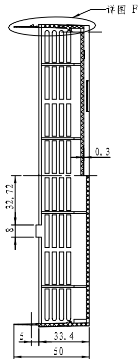
截面 A-A
