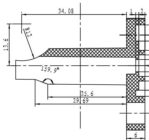
剖面 A-A
