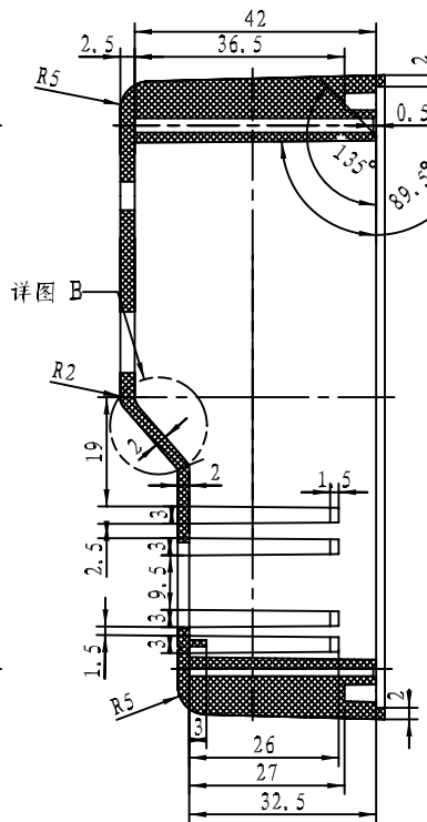
剖面 A-A 技术要求
