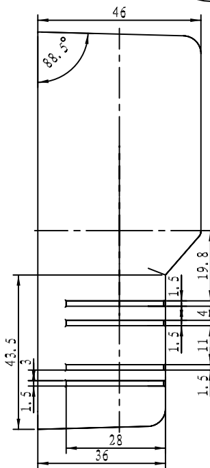
细节 A 比例 4:1
