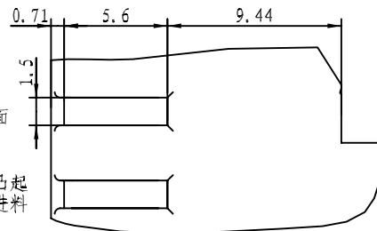
细节 C 比例 4:1
