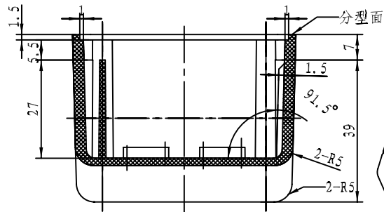
剖面 B-B
