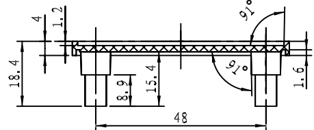
剖面 B-B
