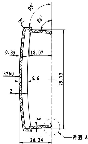
剖面 A-A
