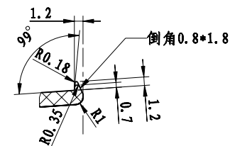
细节 A 比例 2:1
