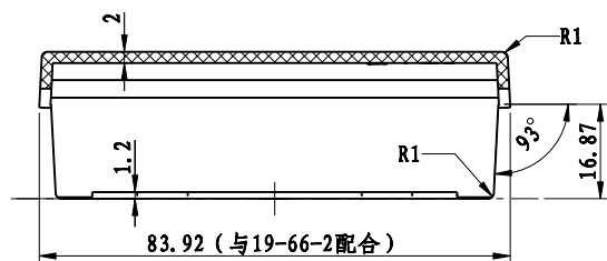
剖面 B-B
