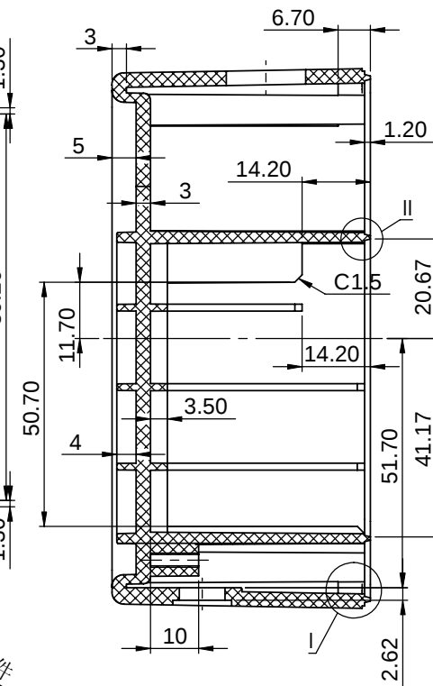
剖面 A-A
