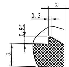
细节 C 比例 5:1
