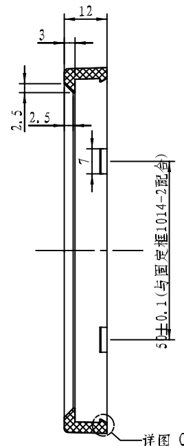
剖面 A-A
