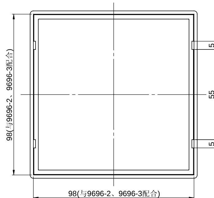
背面(顶杆面)
