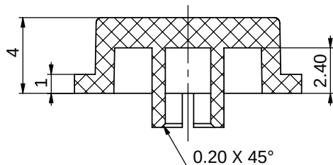
剖面 A-A
