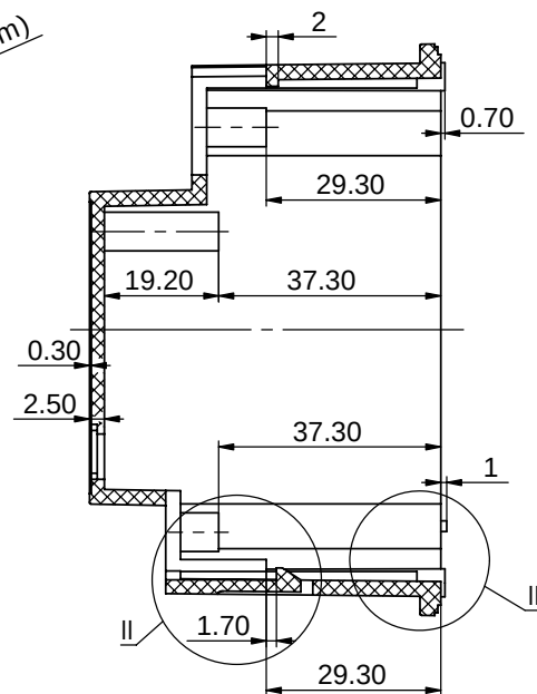
剖面 A-A
