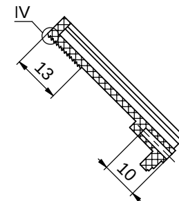
剖面 E-E
