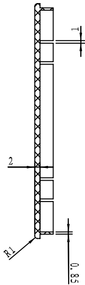
剖面 A-A
