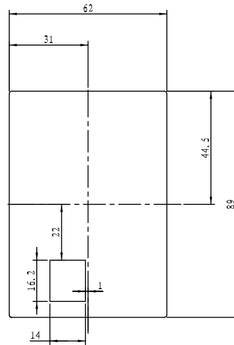
正面、外表面
