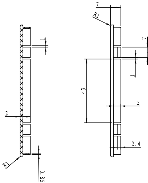
剖面 A-A
