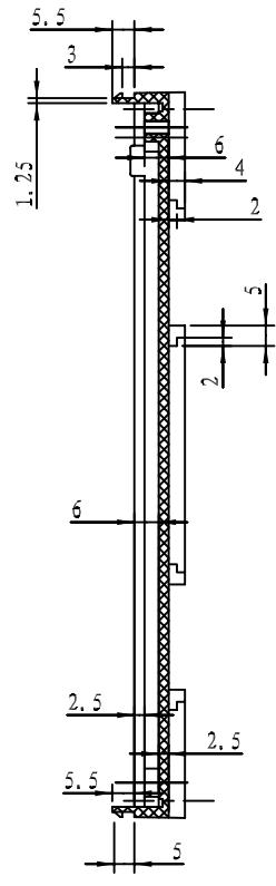
剖面 A-A
