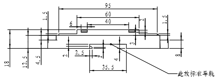
剖面 B-B
