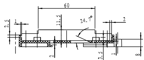
剖面 B-B
