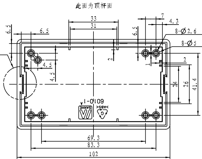
详图 B
