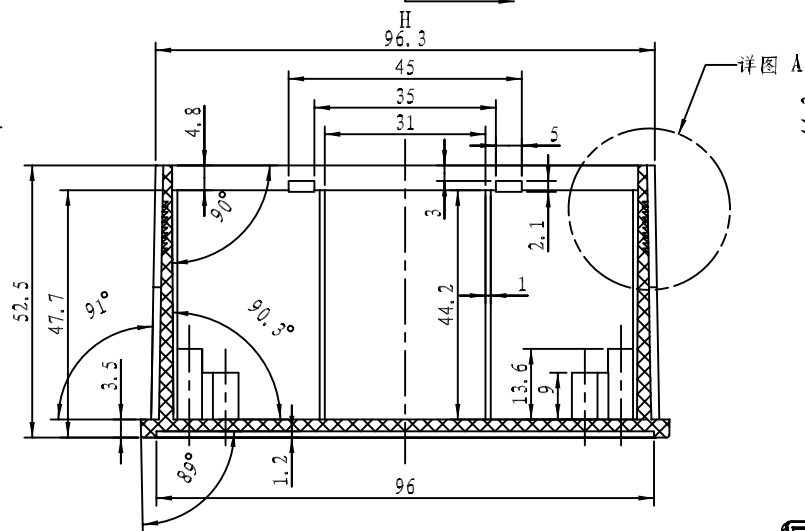
剖面 B-B
