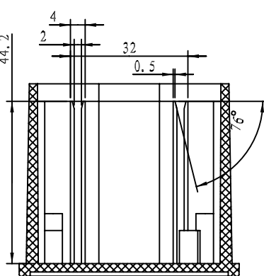
剖面 H-H
