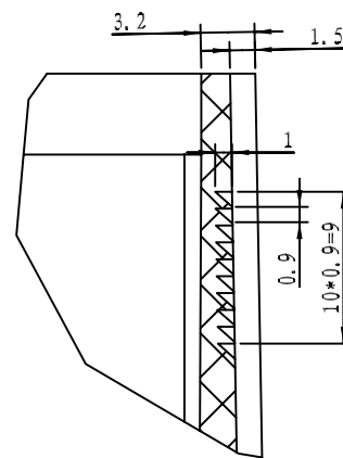
细节 A 比例 3:1
