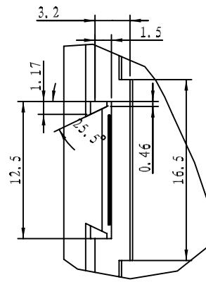
细节 B 比例 3:1
