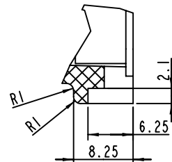
细节 C 比例 2:1
