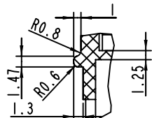
细节 B 比例 2:1
