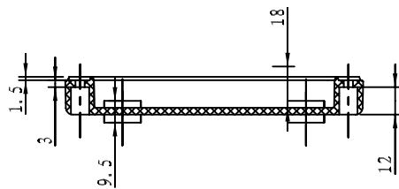
剖面 B-B
