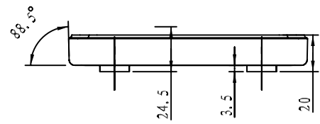
剖面 B-B
