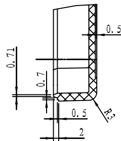
细节 A 比例 1:1
