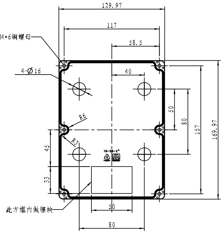
反面 (顶杆放此面)
