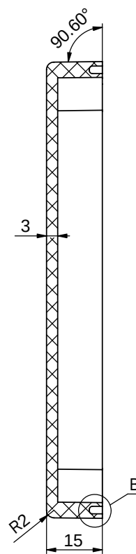
剖面 A-A
