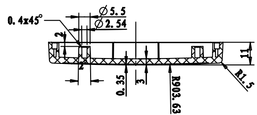
截面 B-B
