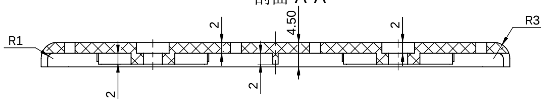
剖面 A-A
