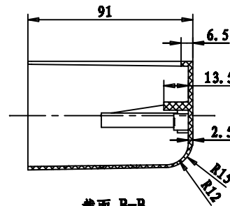
截面 B-B
