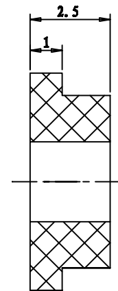
截面 A-A
