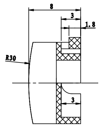
截面 B-B
