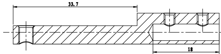
截面 A-A
