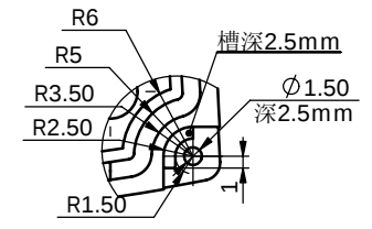
局部视图 G 比例 2:1
