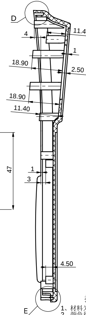
剖面 B-B
