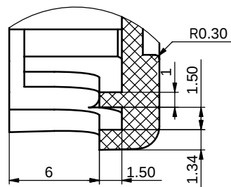
局部视图 E 比例 4:1
