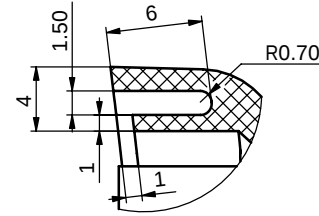
局部视图 D 比例 3:1
