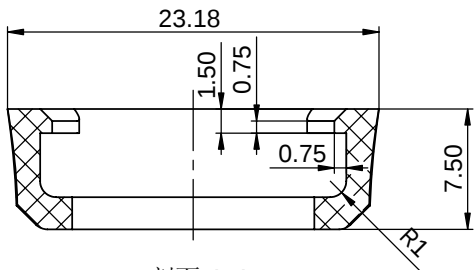
剖面 A-A
